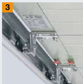
Galets de guidage
